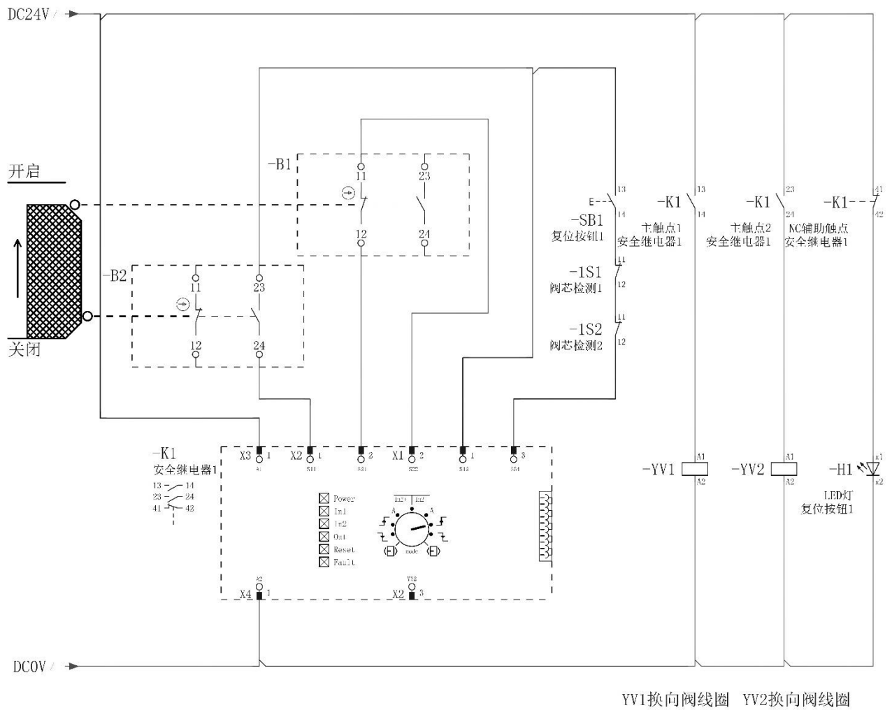
图A.1 电气回路图示例
