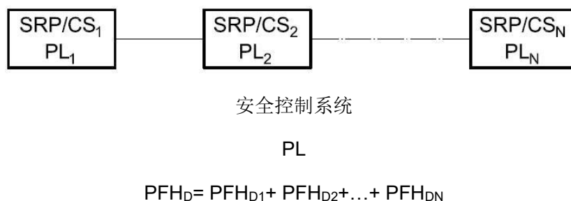
图4 实现总PL的安全控制子系统组合
