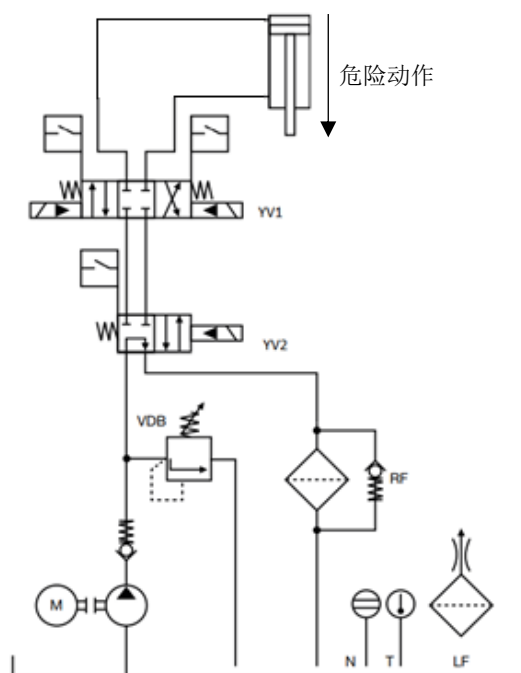
图A.2 液压回路图示例
