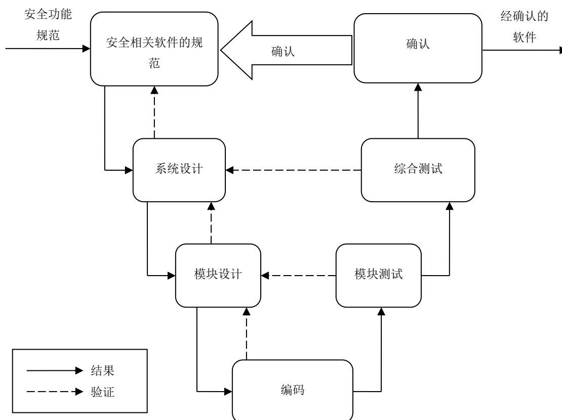
图5 安全相关软件开发用简化V模型
